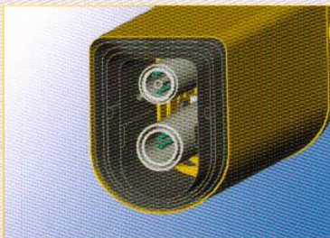
多芯管伸缩油缸，双缸内部沟通，免除了软管卷筒
